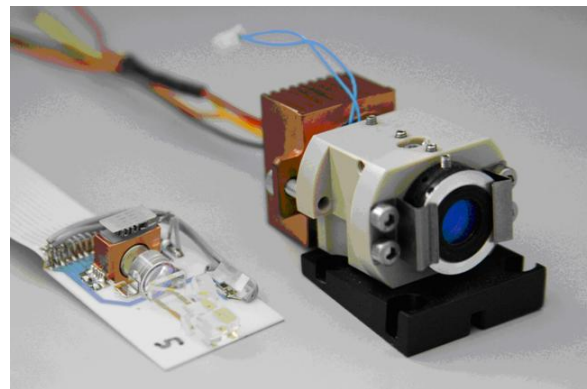
Liniengenerator als Hybrid-Optikmodul und konventionell aufgebautes Laserdiodenmodul
